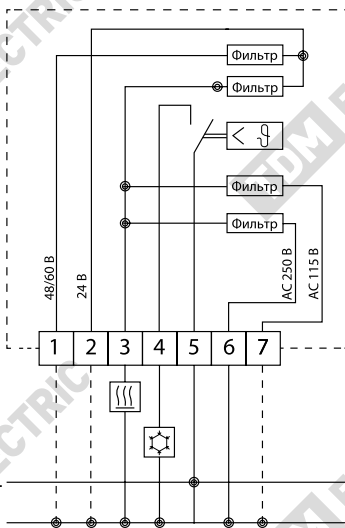
Рисунок 4. Схема подключения вентилятора с термостатом SQ0832-0018
