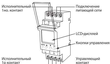
Рисунок 3. Лицевая панель реле
