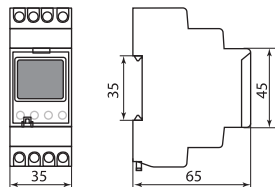
Рисунок 1. Габаритные и установочные размеры реле, мм
