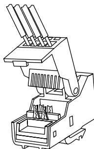
Рисунок 4. Расположить провода в джеке согласно разметке.
