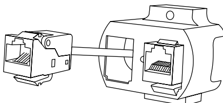
Рисунок 6. Вставить джек в суппорт.
